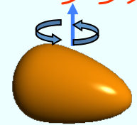
クラスター構造
