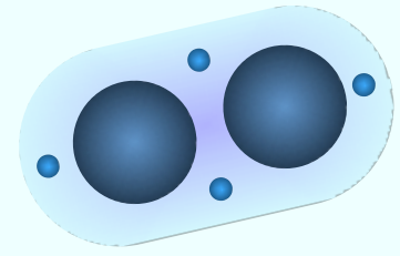
クラスター構造
