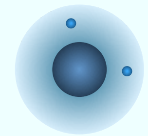
中性子ハロー
