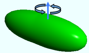
ハイパー変形
